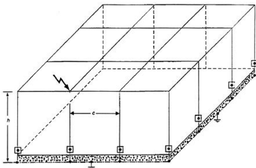
Hình C.1 - Giá trị hệ số k_c trong trường hợp hệ thống thu sét là dây
