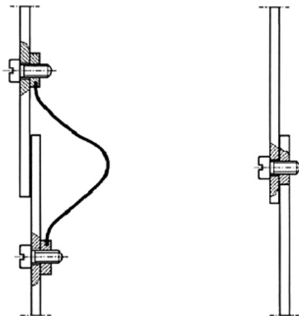
Hình E.35a - Cầu nối bằng đai kim loại linh động
