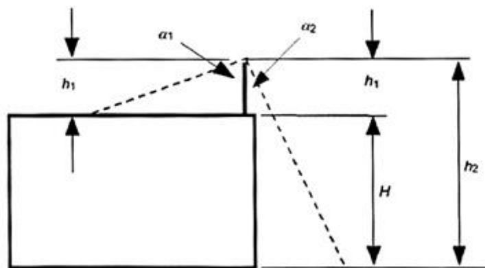
Hình A.1 - Không gian được bảo vệ bởi thanh thu sét thẳng đứng
