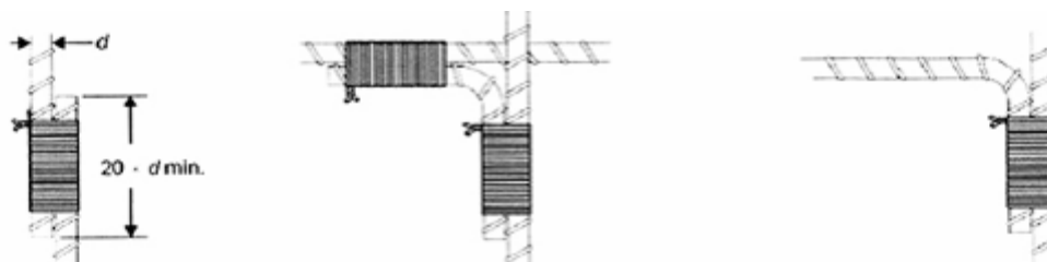
Hình E.5b - Các mối ghép được kẹp theo IEC 62561 sau này (phù hợp với dòng sét và các mục đích EMC)
