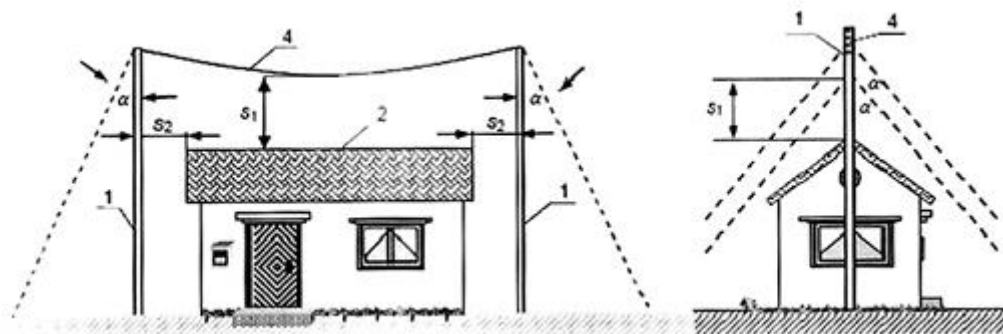
Hình E.14a - Hình chiếu đứng song song với mặt phẳng chứa hai cột
