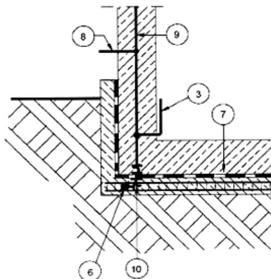
Hình E.40c - Kết nối từ điện cực đất móng tới cốt thép dẫn qua màng chống ẩm
