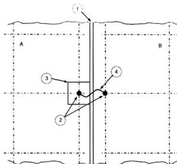
Hình E.11a - Lắp đặt các dây dẫn liên kết trên các tấm bê tông cốt thép đúc sẵn bằng liên kết dây dẫn bắt vít hoặc hàn
