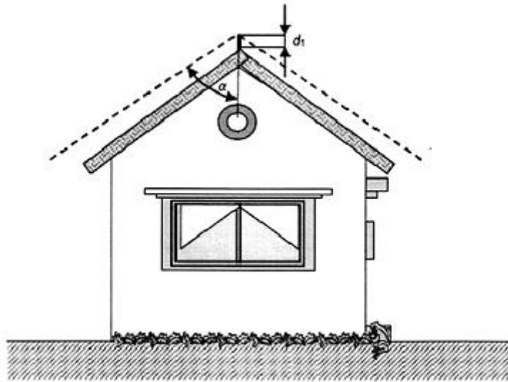
Hình E.16b - Hình chiếu đứng vuông góc với mặt phẳng có chứa dây dẫn
