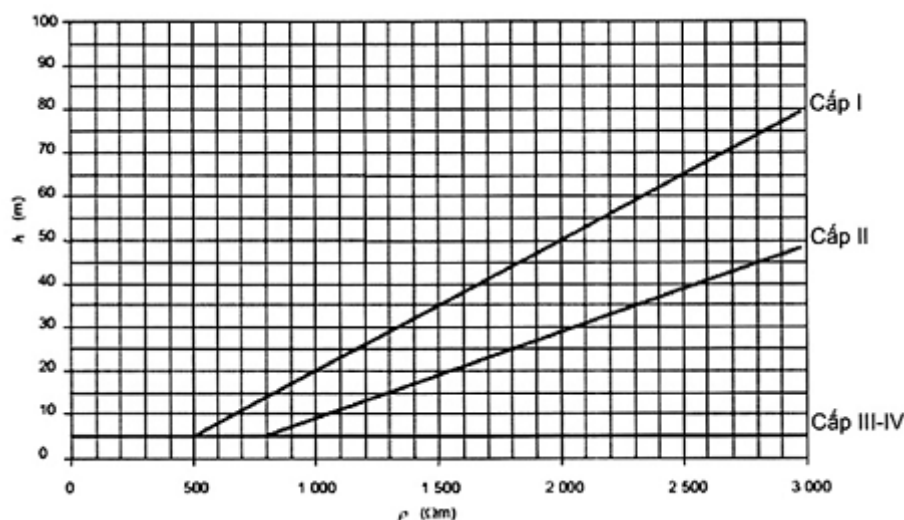
Hình 3 - Chiều dài nhỏ nhất của từng điện cực đất theo cấp LPS
