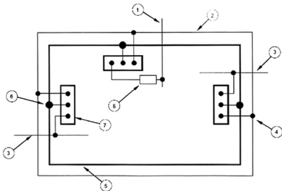
Hình E.45 - Ví dụ về liên kết trong trường hợp các lối vào đa điểm của các bộ phận dẫn điện bên ngoài và một đường dây điện hoặc viễn thông sử dụng dây dẫn vòng bên trong cho kết nối với nhau của các thanh liên kết
