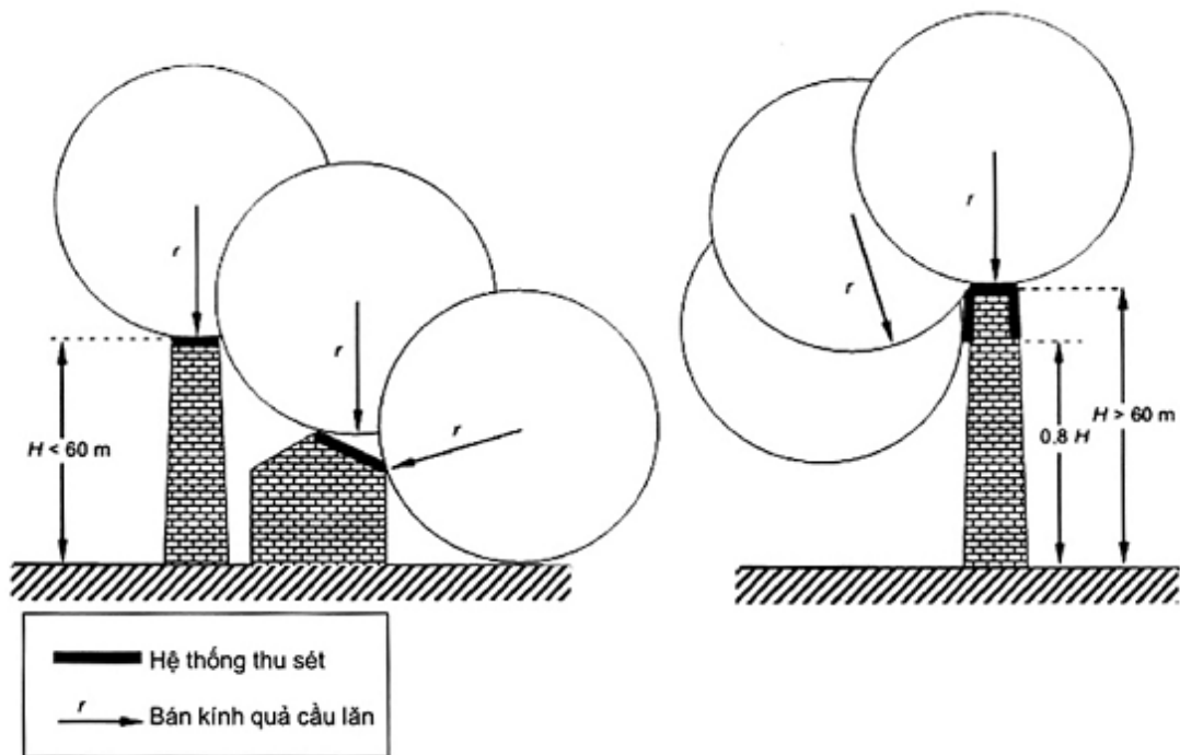
Hình A.6 - Thiết kế hệ thống thu sét theo phương pháp quả cầu lăn
