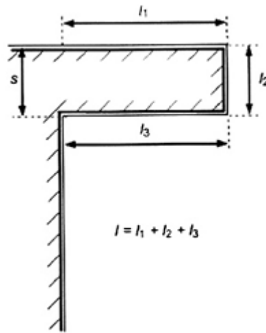
Hình 2 - Vòng kín trong dây dẫn sét
