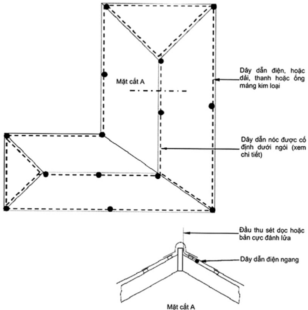
Hình E.22 - Bốn ví dụ chi tiết về một LPS trên kết cấu có mái lợp ngói nghiêng
