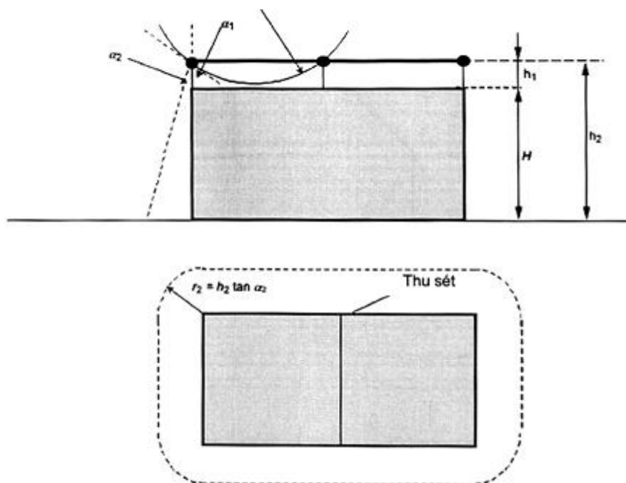
Hình A.4 - Không gian được bảo vệ bởi các dây cách ly kết hợp trong lưới theo phương pháp góc bảo vệ và phương pháp quả cầu lăn
