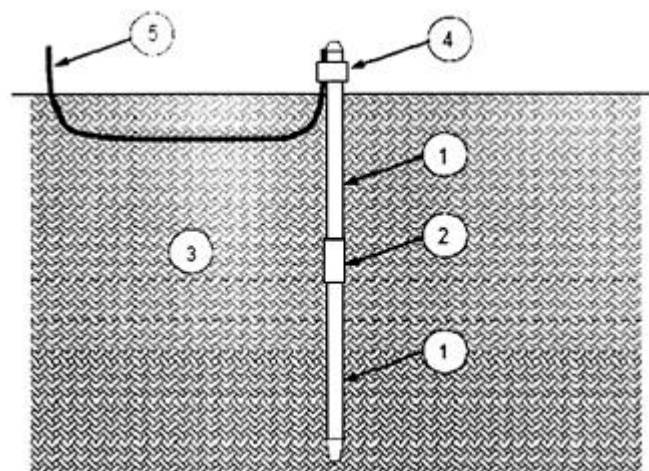
Hình E.41a - Ví dụ về sắp xếp nối đất loại A có điện cực kiểu dây dẫn dọc
