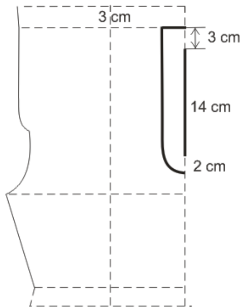
Hình 2.5 Miệng túi, lót túi
