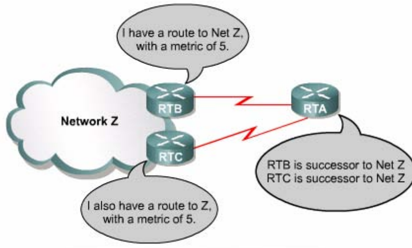
Hình 3.2.6.b. RTA có thể cài đặt nhiều đường successor nếu chúng có cùng chi phí
