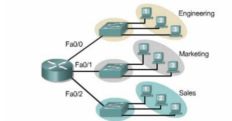
Hình 8.1.2.a.3 miền quảng bá trên 3 switch khác nhau.
