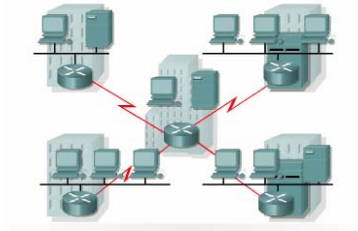
Hình 2.3.1.a. Mạng WAN trước đây và hiện nay.
