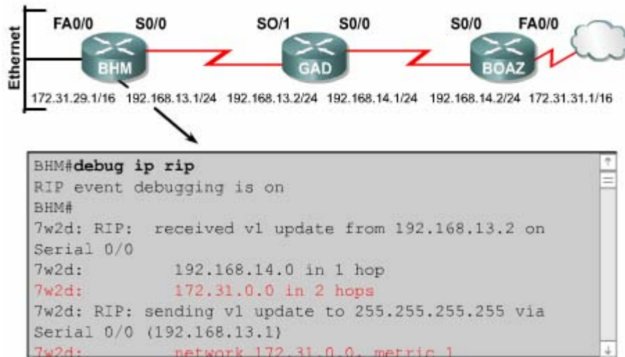
Hình 7.2.6c: Trùng Subnet
