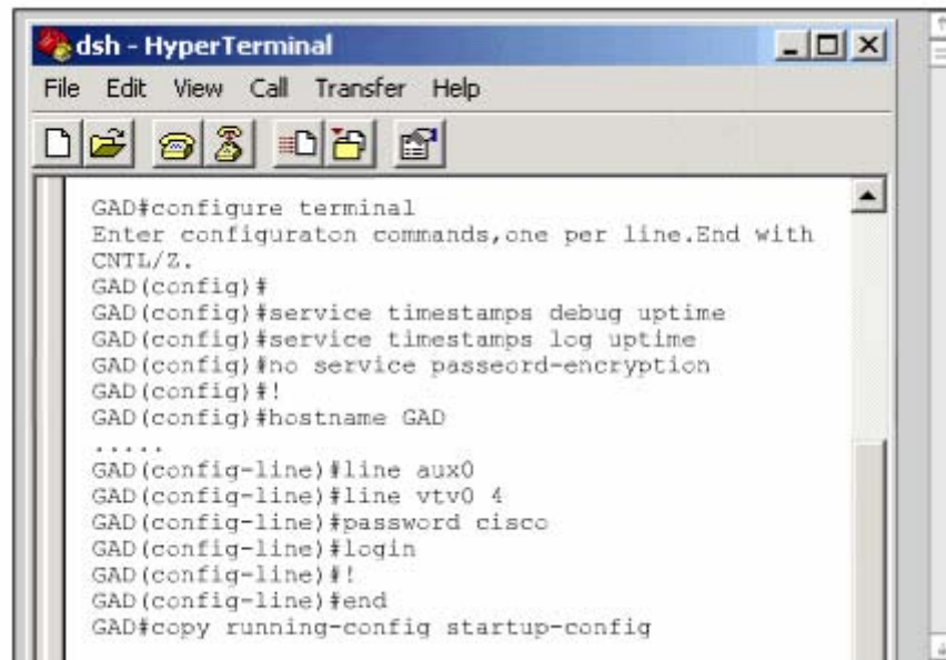
Hình 5.2.4b: Quá trình chép tập tin cấu hình vào router bằng kết nối HyperTerminal
