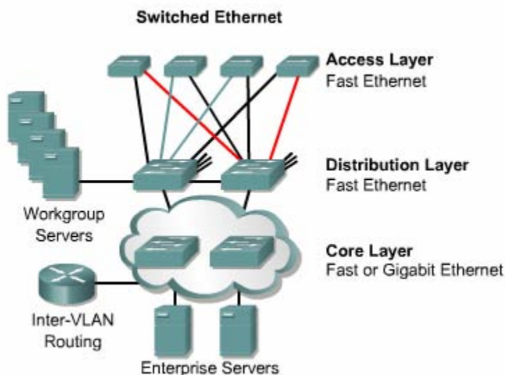
Hình 8.2.1.b VLAN từ đầu cuối- đến - đầu cuối.
