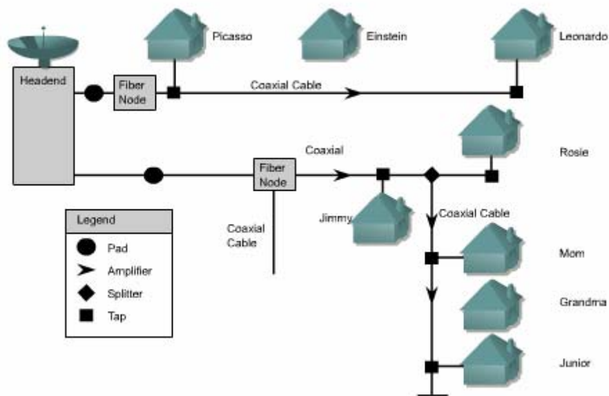
Hình 2.2.8.a. Cable modem
