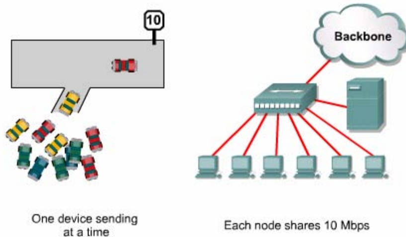
Hình 4.1.1.a.Kết nối user dùng Hub.Các user trên cùng một Hub truy suất cùng một băng thông đường truyền cũng giống như nhiều xe hơi cùng rẽ vào một làn đường vậy.Con đường này chỉ có một làn đường nên tại một thời điểm chỉ được một xe rẽ mà thôi.
